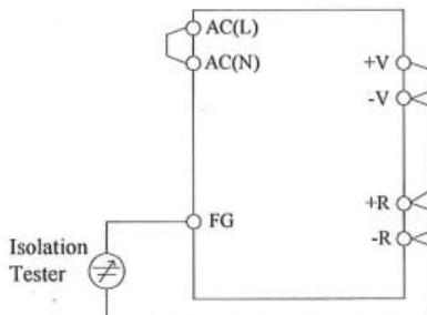
( B ) HWS50A
