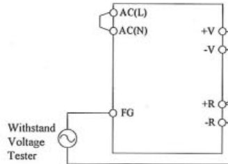
( B ) HWS50A
