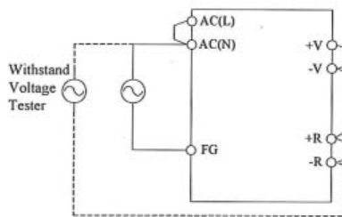
( B ) HWS50A
